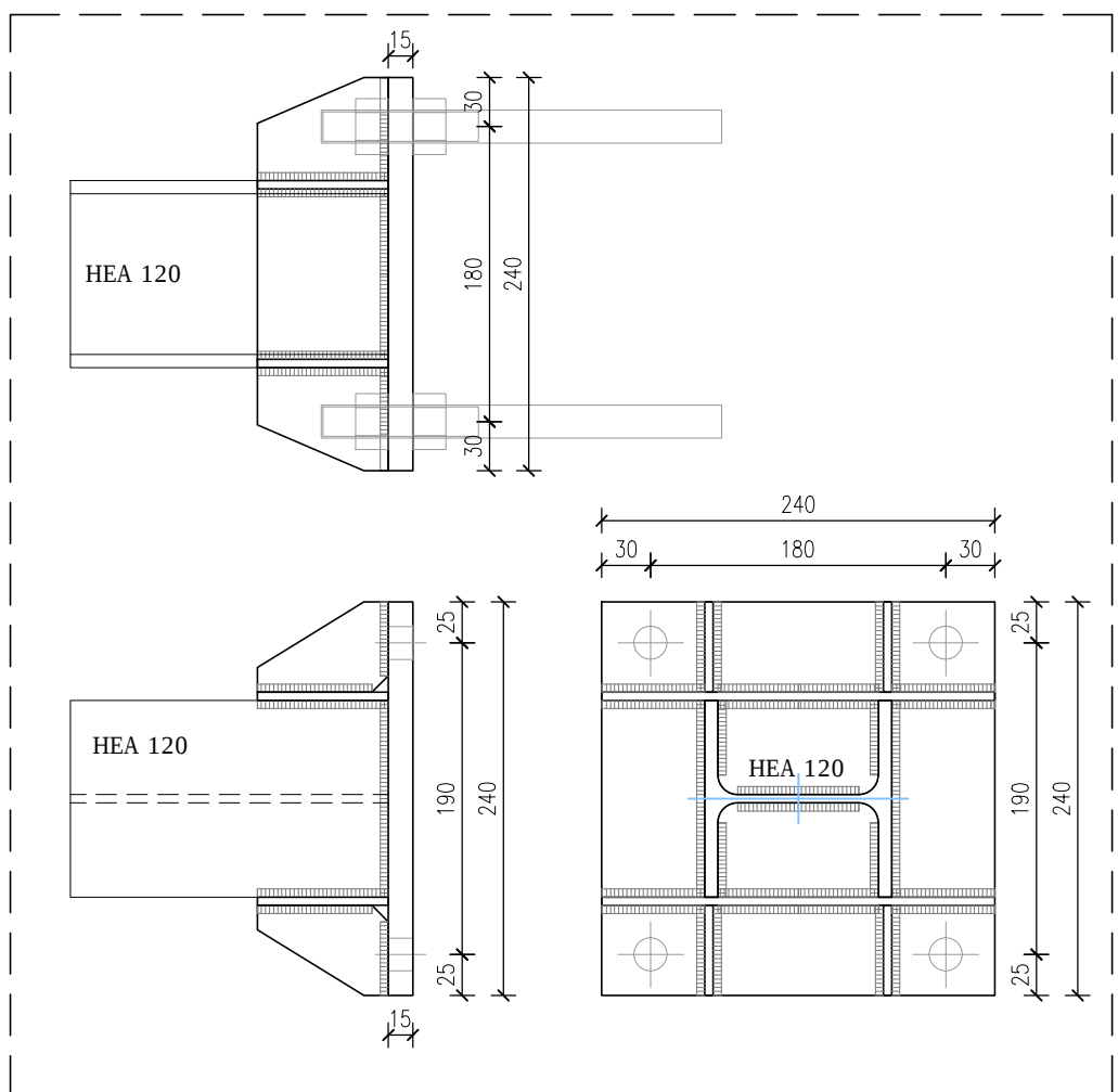
Particolare Piastra "A" scala 1:5
