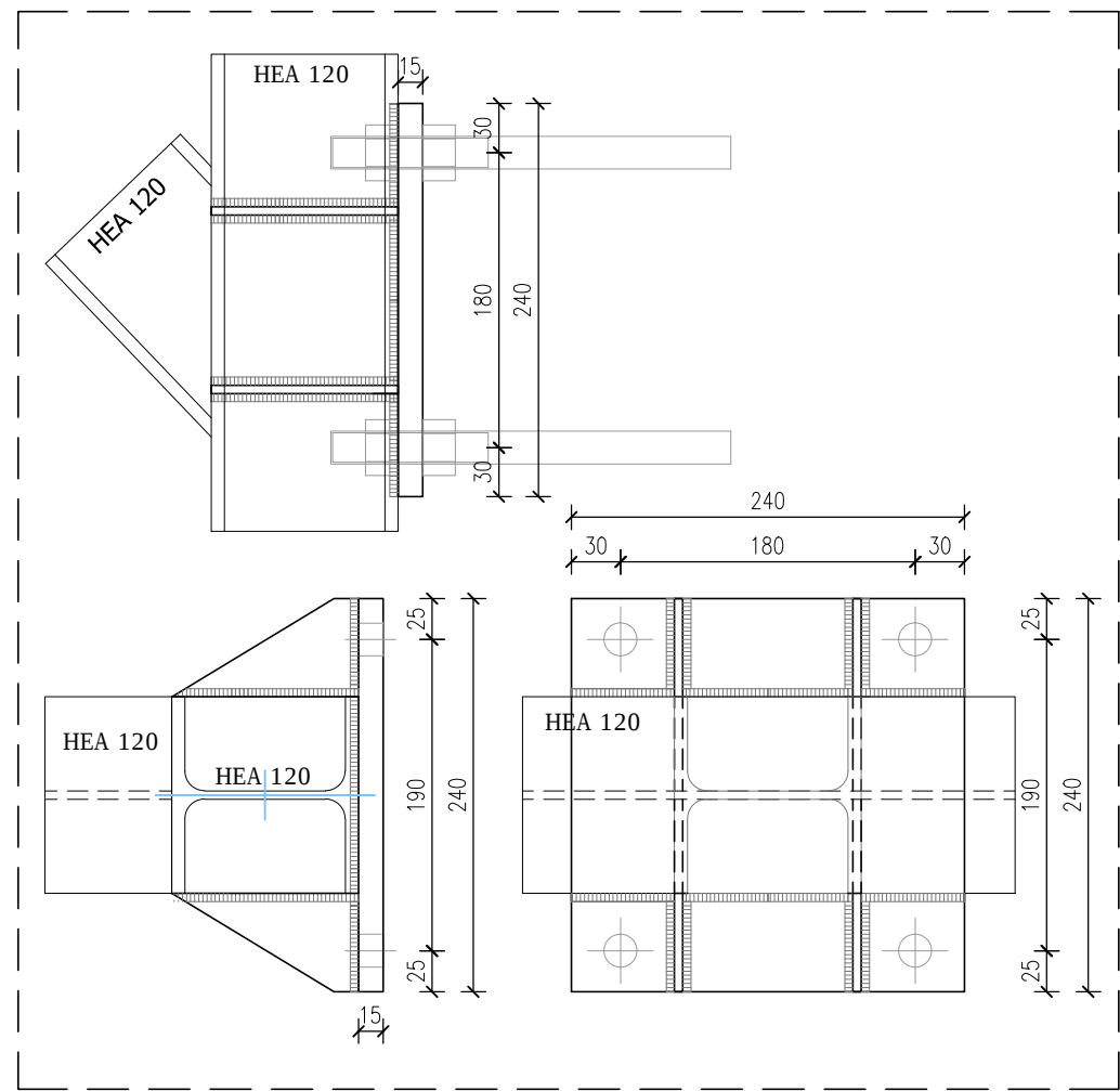
Particolare Piastra "B" scala 1:5
