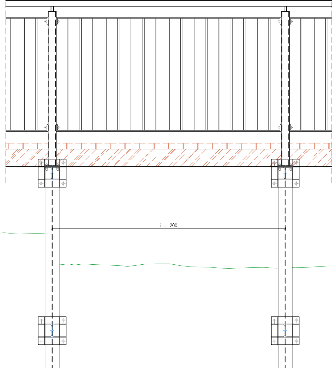
Particolare - Balaustra di protezione in progetto scala 1:20
