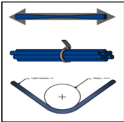
INSTALLAZIONE CORRETTA
